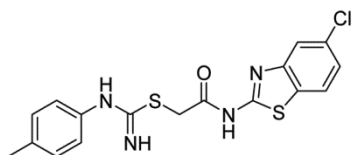
N-(5-Chloro-benzothiazol-2-yl)-2-p-tolylcarbamimidoylsulfanyl-acetamide (27)
